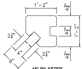
45° PILASTER 158 lbs./ft.
